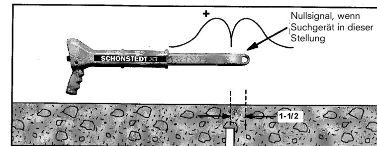
Abb. 17 Signalverlauf bei waagrecchter Suchgerätstellung
