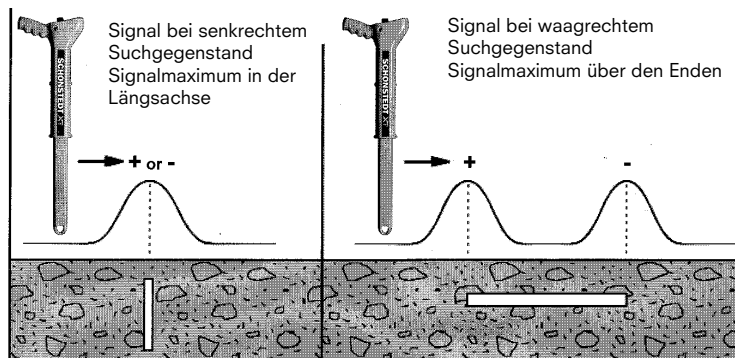
Abb. 6 Signale von senkrechten und waagrecchten Gegenständen
