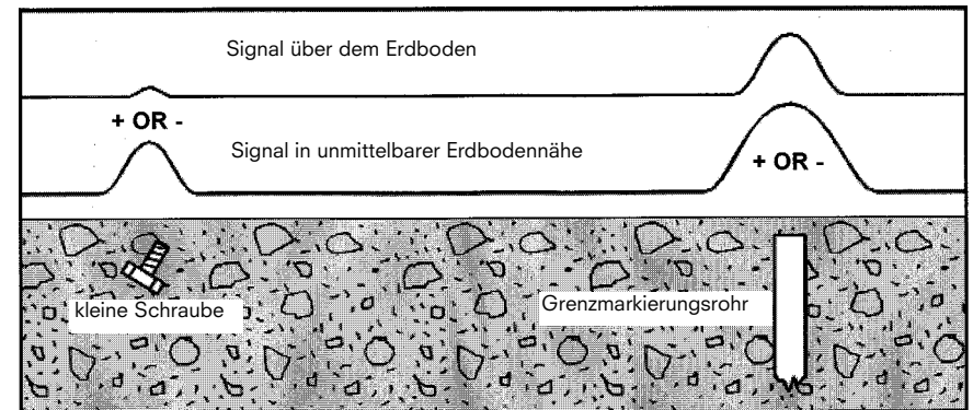
Abb. 8 Anheben des Suchgerätes eliminiert unerwünschte Signale
