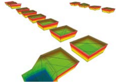
Volumenberechnung von Fundamenten
