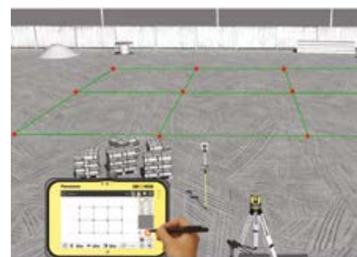
Abstecken eines Rasters im Außenbereich
